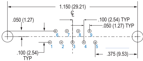
9 SOCKET M83513/25-A
