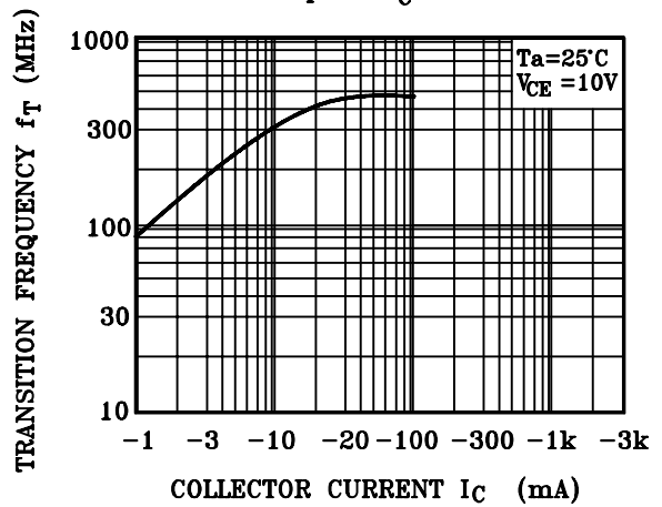
f_T - I_C
