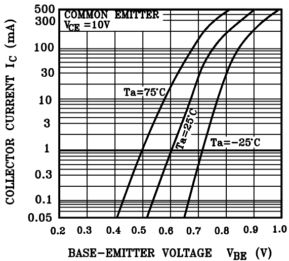
I_C - V_{BE}
