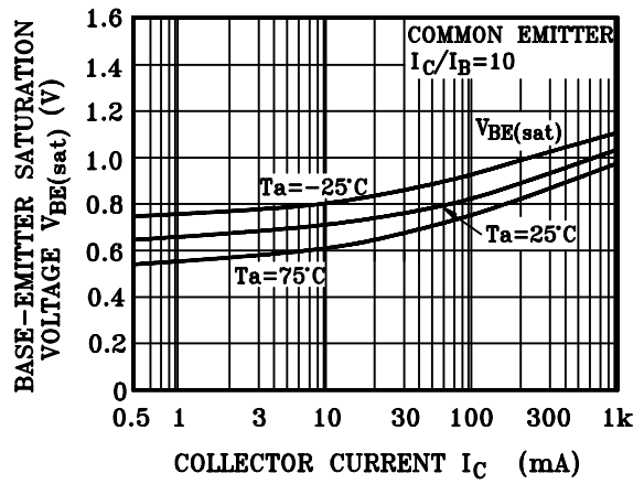
V_{BE(sat)} - I_C
