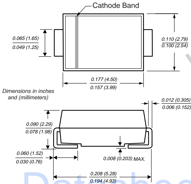
DO-214AC (SMA)
