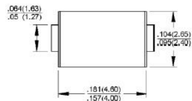
DO-214AC (SMA)
