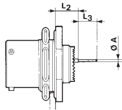
receptacle type 7
