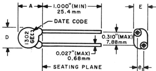
DIMENSIONS TABLE
