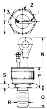
STUD TYPE 1
