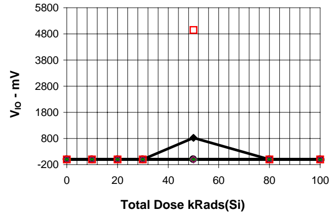
V_{IO} ; V_+=5V , V_{CM}=0V , AMP 2 vs Total Dose
