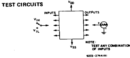
Fig. 10 - Input voltage.
