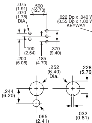
Horizontal Actuation
